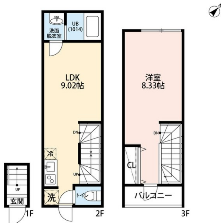
【間取り図】
